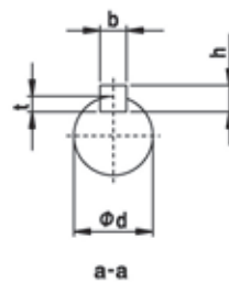
a-a Output shaft
